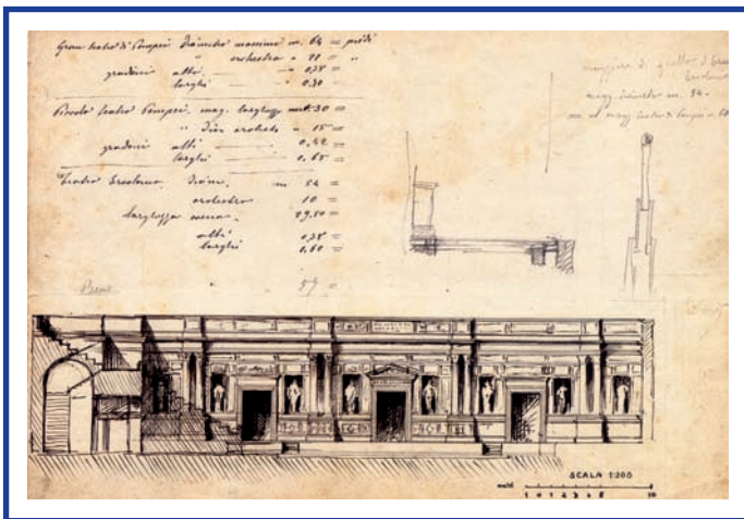
Ricostruzione della Frons Scenae del Teatro Romano eseguita da G. Vacchetta
