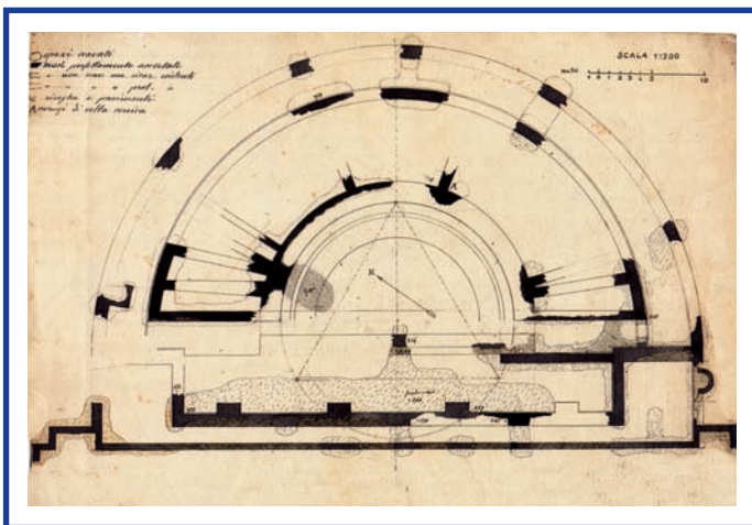
Pianta del Teatro Romano eseguita da G. Vacchetta
